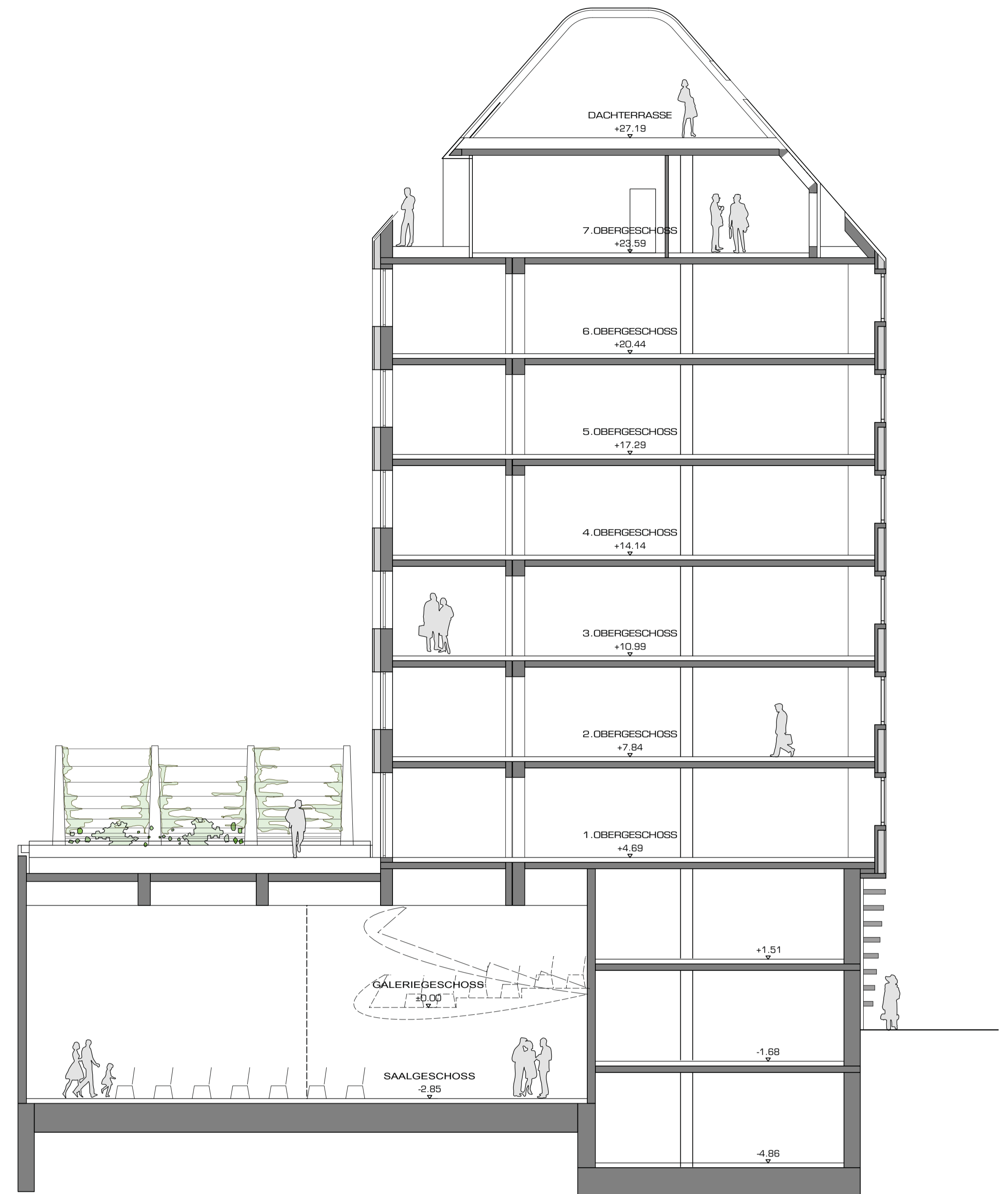
SCHNITT BB M 1:100
