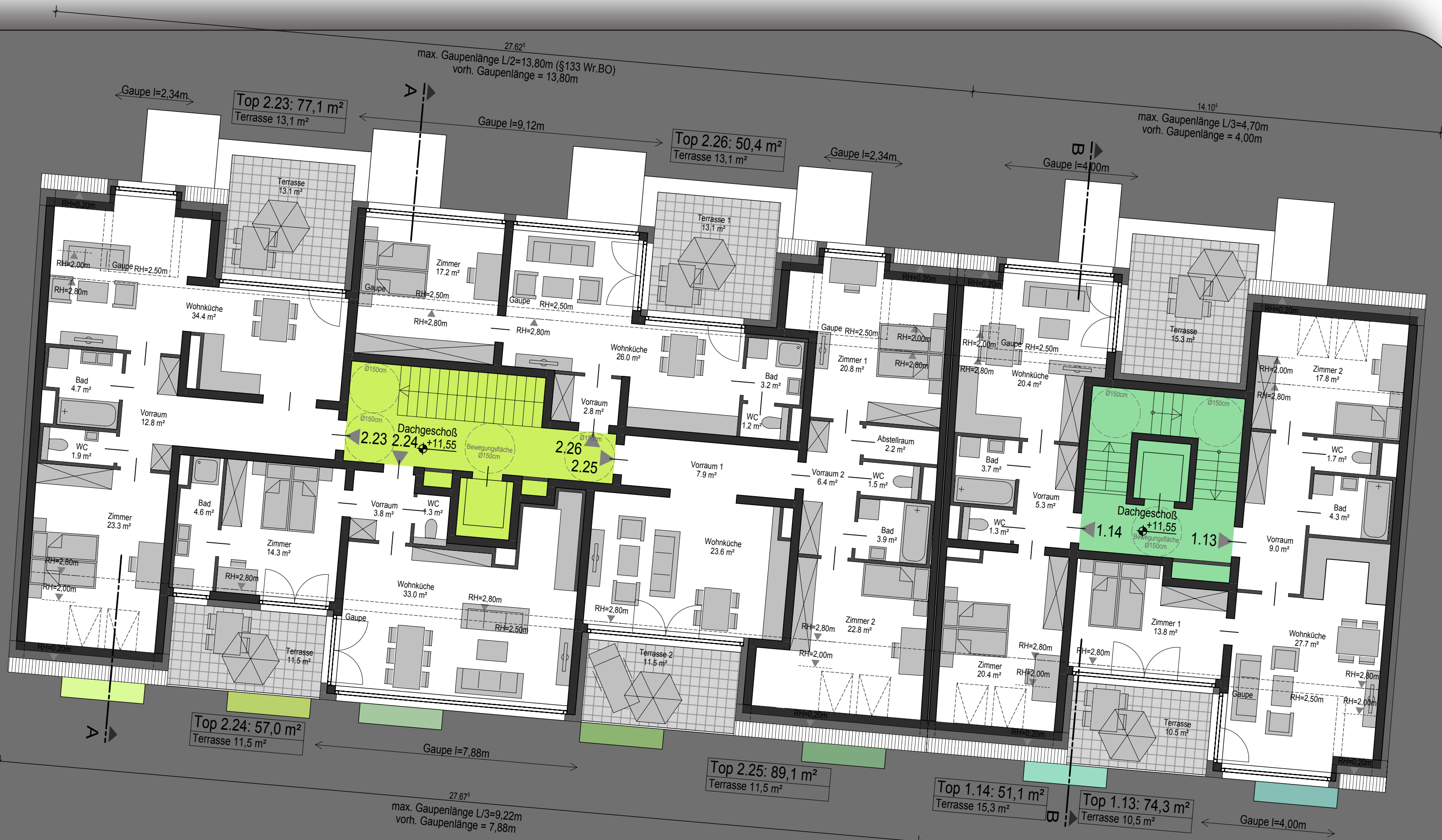
GRUNDRISS DG
